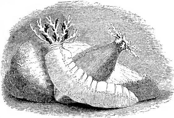
SEA-CUCUMBERS ( Holothuria ).
